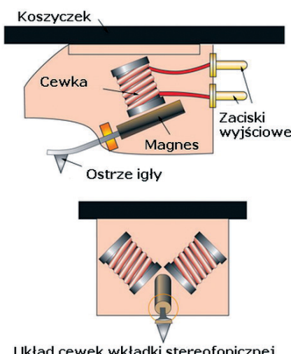
Układ cewek wkładki stereofonicznej
