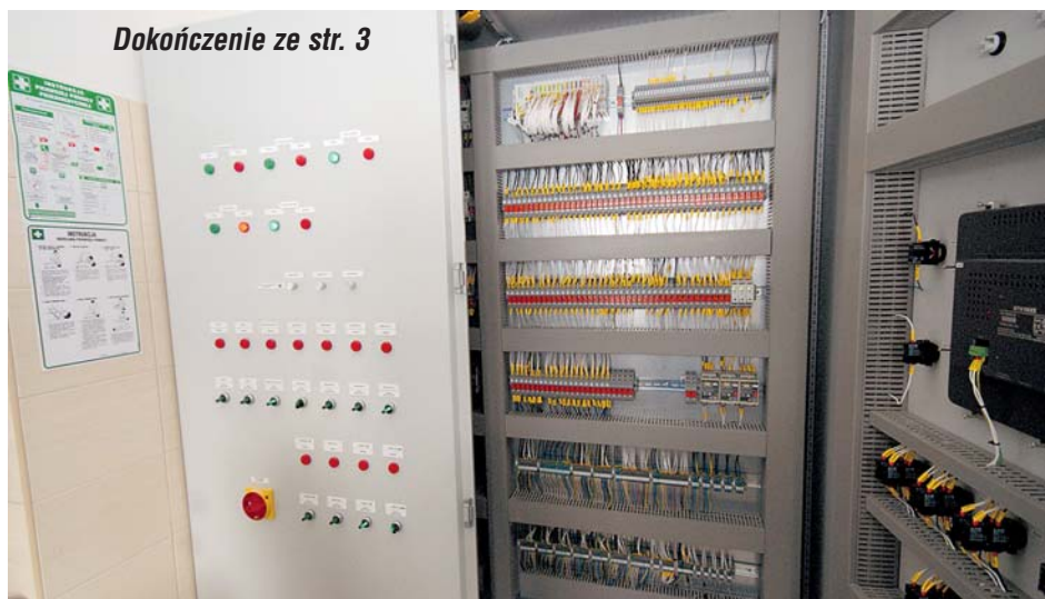
Szafa sterownicza - główny mózg oczyszczalni.
